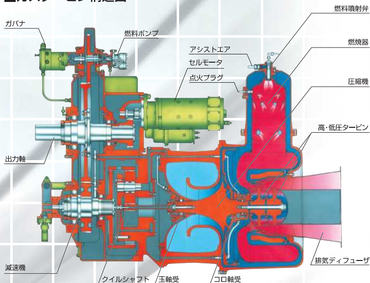
■ガスタービン構造図
